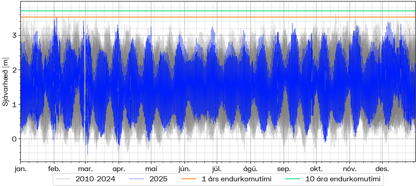
Landeyjahöfn - Sjávarhæðamælingar 2025
