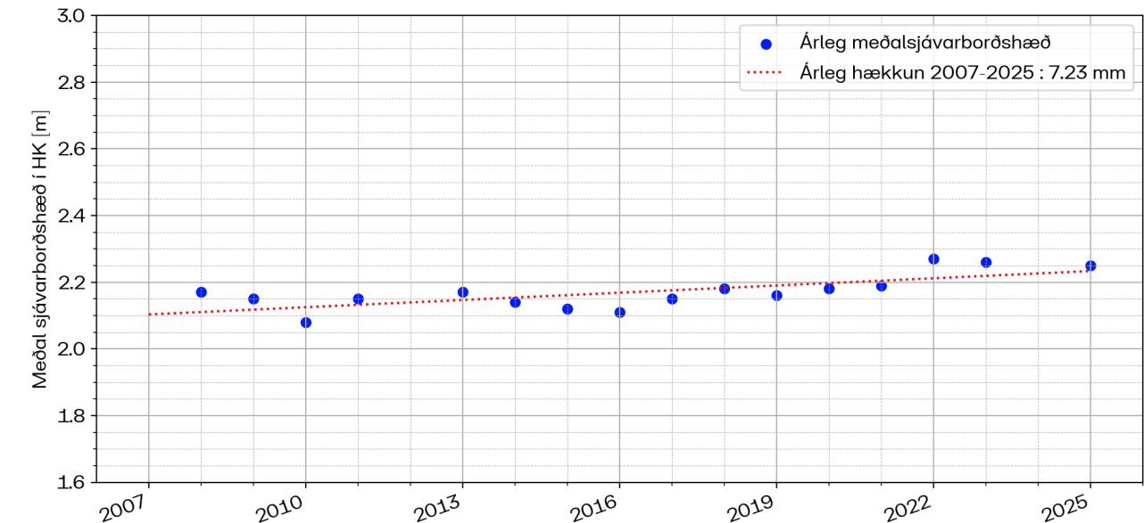
Akranes - Meðal sjávarborðshæð
