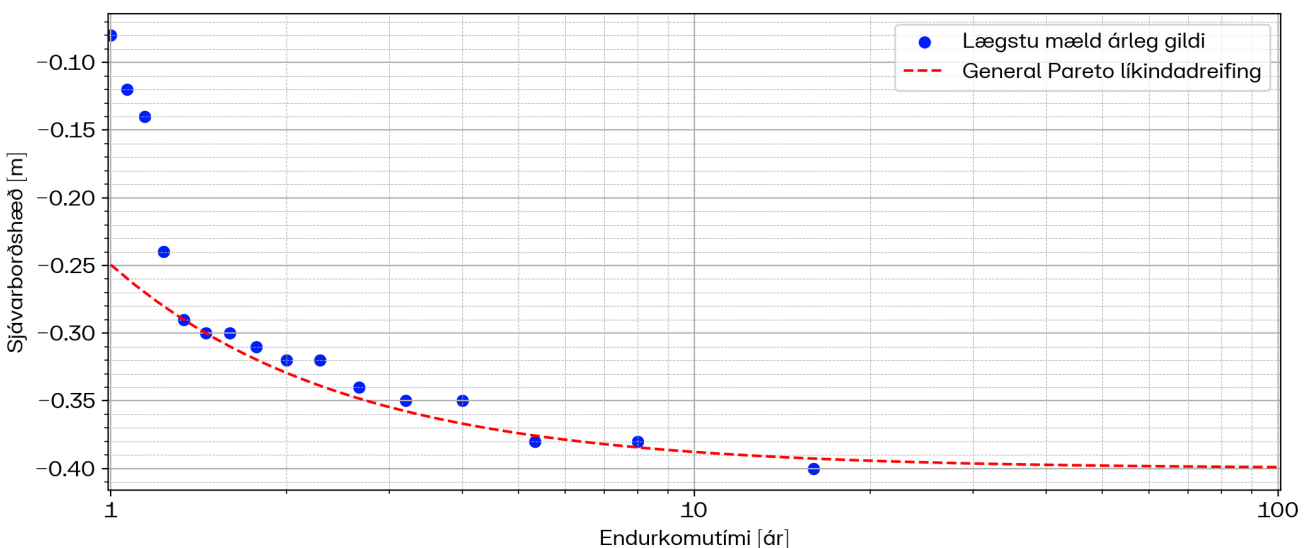
Akranes - Minnsta árlega sjávarborðshæð
