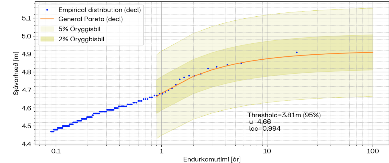
Akranes - Endurkomutími sjávarhæðar
