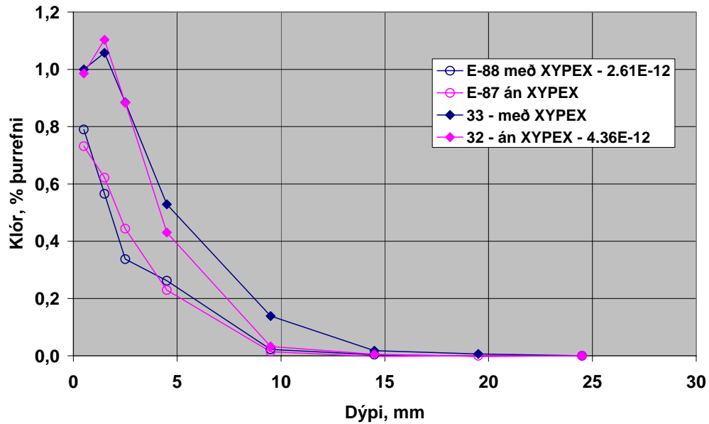
Mynd 29. Niðurstöður úr NT Build 443 prófun.
