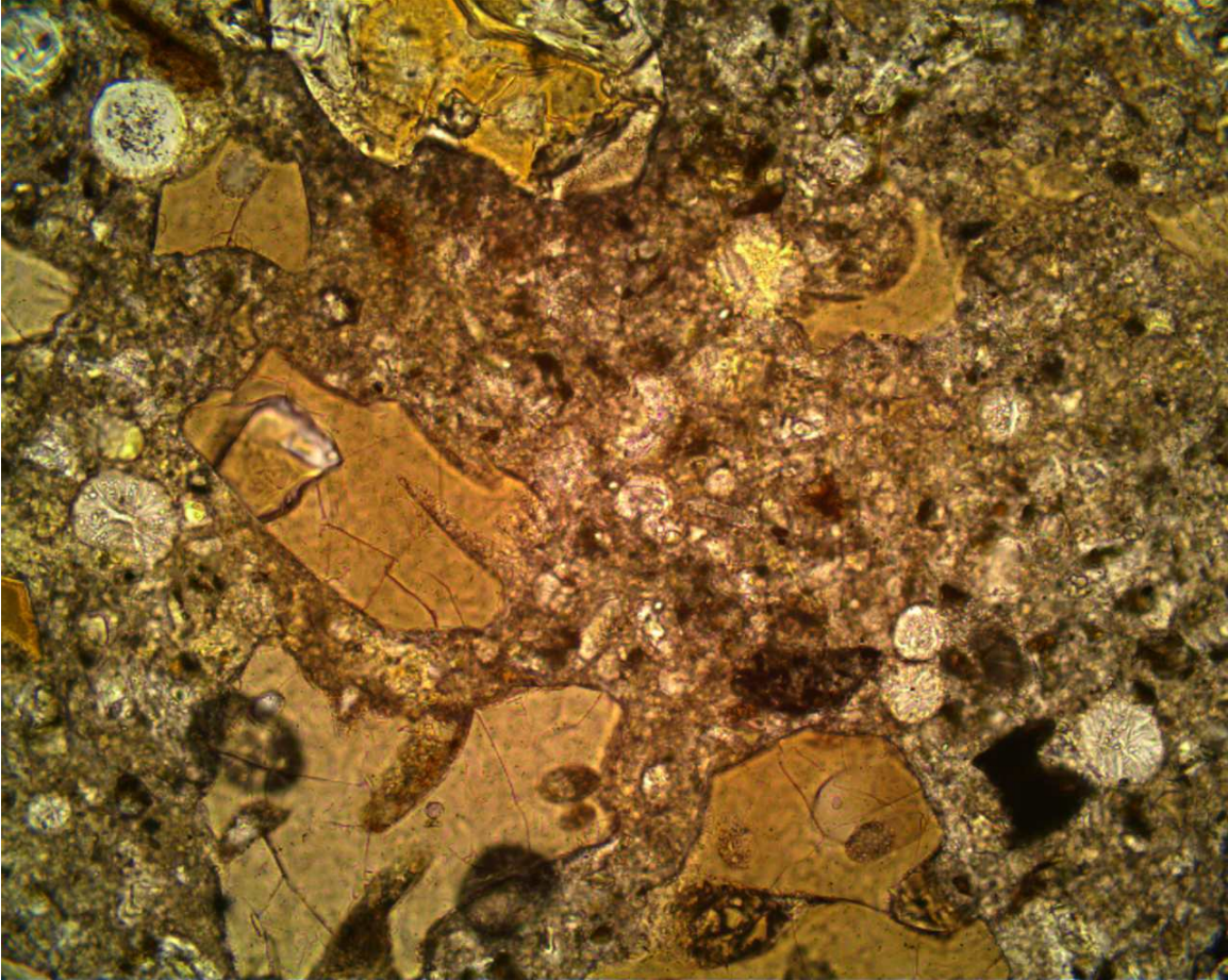
Mynd 6. Útfellingar í holrými í steinsteypu við yfirborð. Holrýmin eru frá 25 til 60 míkron í þvermál. Myndin er tekin í 20x stækkun (0,714 x 0,495 mm)
