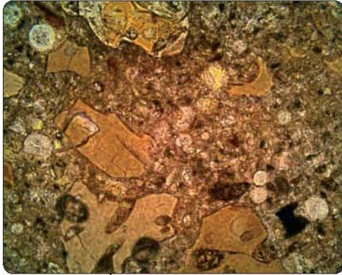
Breiðabalakvísl við Kirkjubæjarklaustur. Smásjármýnd úr steypunni í brúnni yfir Breiðabalakvísl. Myndast hafa hringlaga XYPEX-kristallar í holrýmum þar sem áður var vatn. Stækkun myndar er 20-föld.
