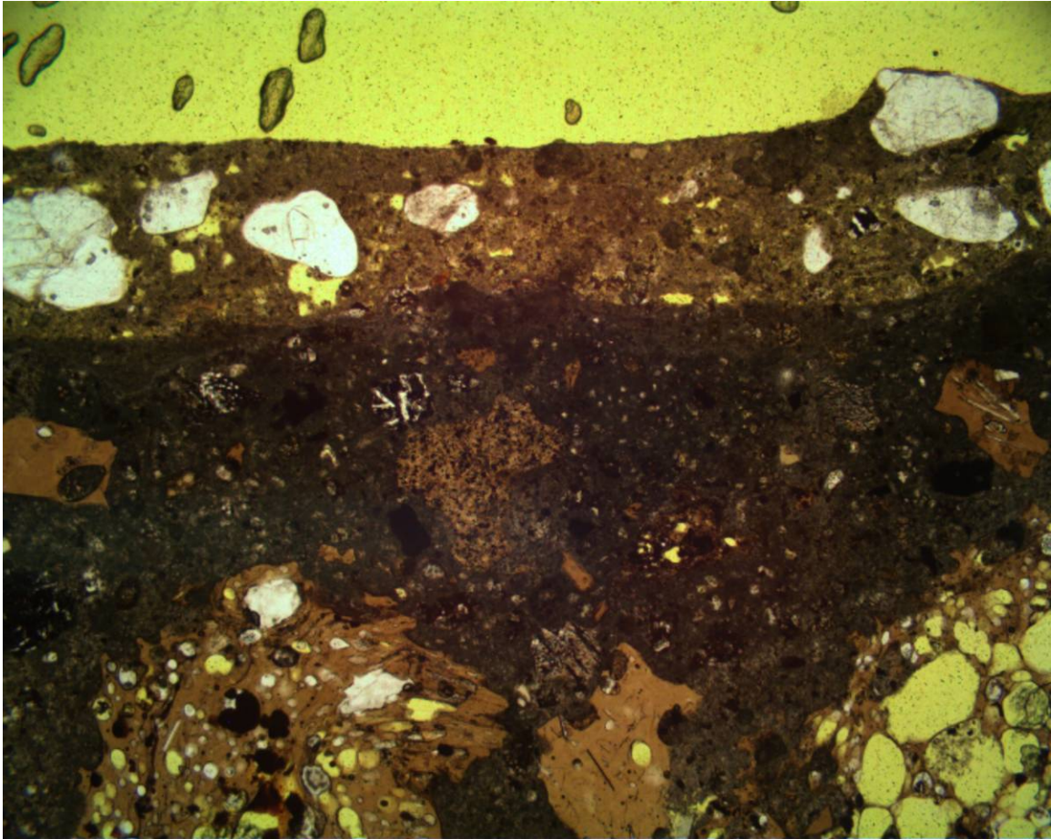
Mynd 13. Sýni með XYPEX concentrate lagi í yfirborði í steypunni úr Tungná. Myndin er tekin í 5x stækkun..
