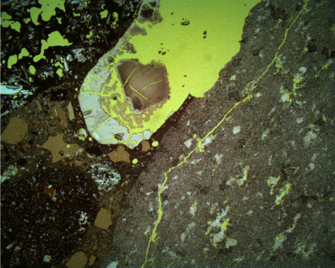
Mynd 12. Alkalívirkt líparít á um 25 mm dýpi er líparít.
