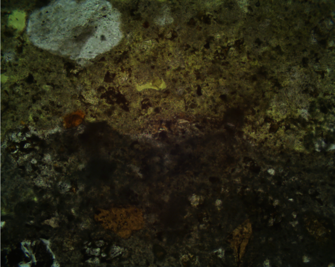
Mynd 14. XYPEXið loðir mjög vel við steypuna. Myndin er tekin í 20x stækkun..
