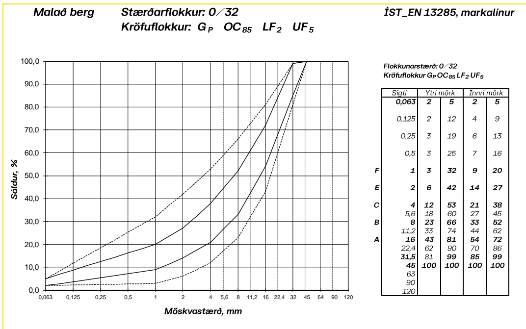
Mynd 5-12: Markalínur fyrir malað 32 mm berg í burðarlag
