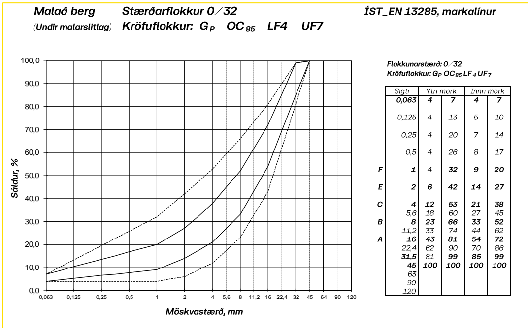
Mynd 5-18: Markalínur fyrir 32 mm malað berg í burðarlág malarvega
